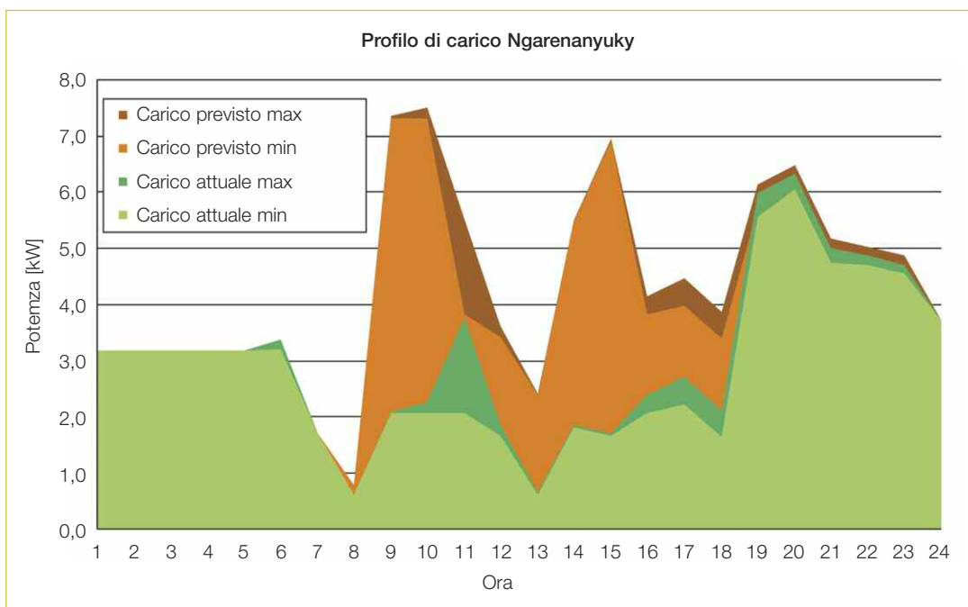
Figura 7 L'immagine riporta una stima delle curve di carico attuali (tonalità verdi) e previsto (tonalità marroni). La differenza all'interno di una tonalità rende ragione del fatto che alcuni carichi vengono attivati saltuariamente.
