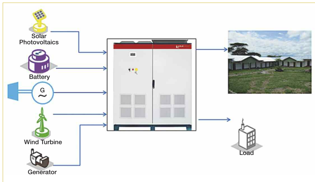
Figura 1 Rappresentazione della micro-grid con particolare riferimento all'Interface Converter.
