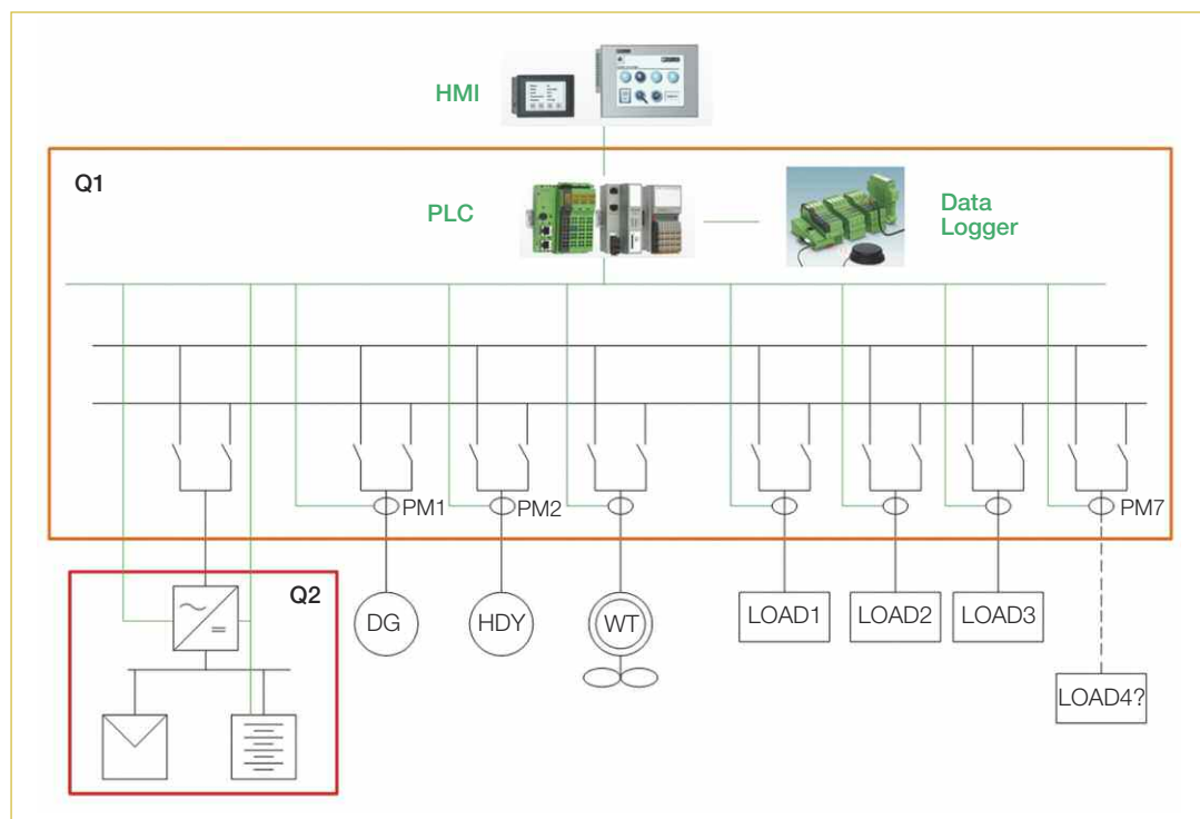
Figura 8 Rappresentazione schematica dell'impianto della micro-grid.
